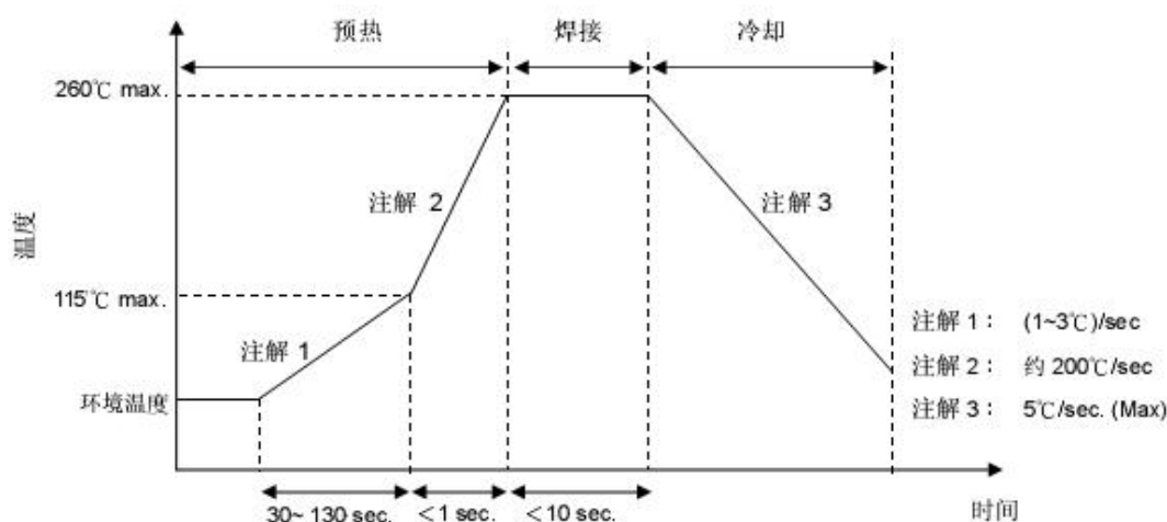
波峰焊曲线
